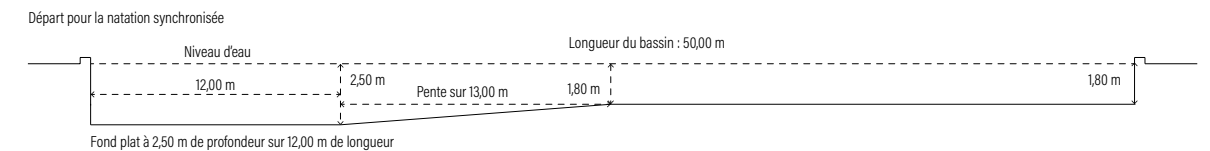
Coupe schématique d'un bassin de type GE*
