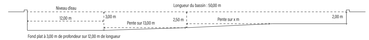
Coupe schématique d'un bassin de type GE*
